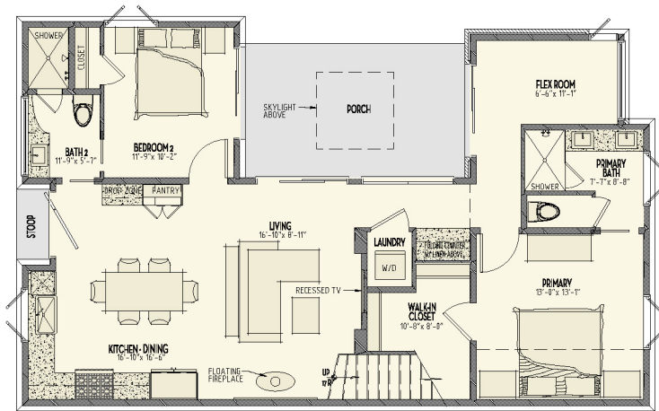
FIRST FLOOR SCALE: 1/8" = 1'-0"
